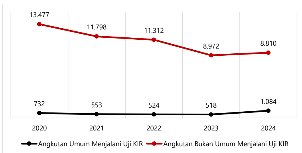
Gambar 6.5 Jumlah Angkutan Umum dan Angkutan Bukan Umum Menjalani Uji KIR di Kabupaten Klaten Tahun 2020-2024
