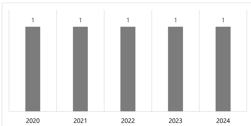
Gambar 6.6 Jumlah Stasiun Kereta Api di Kabupaten Klaten Tahun 2020-2024
