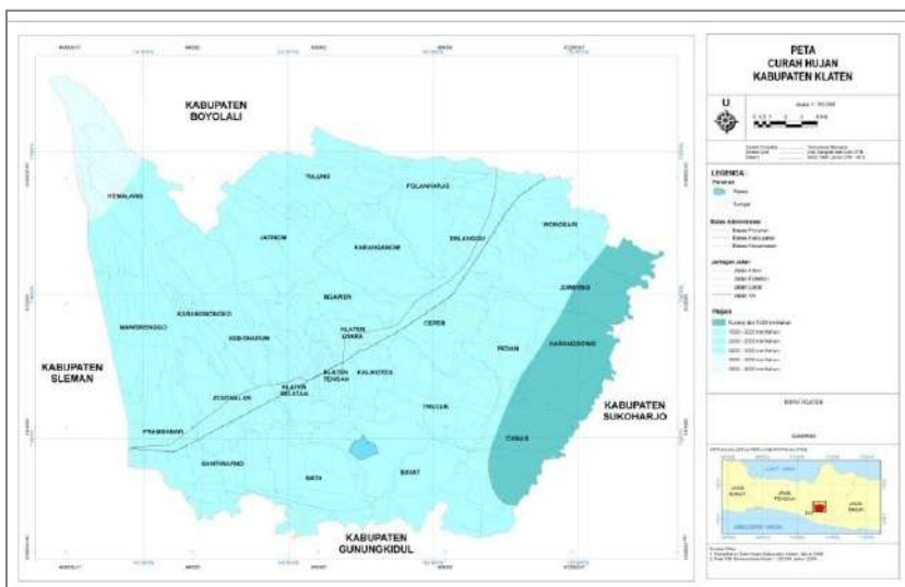
Gambar 2.6 Peta Klimatologi Kabupaten Klaten Sumber: RTRW Kabupaten Klaten 2021-2041
