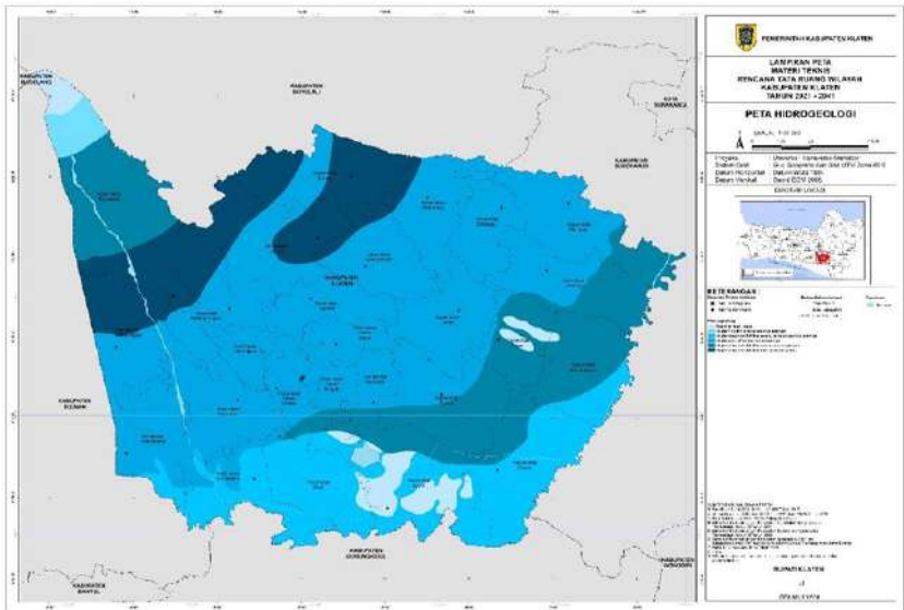
Gambar 2.7 Peta Hidrogeologi Kabupaten Klaten Sumber: RTRW Kabupaten Klaten Tahun 2021-2041
