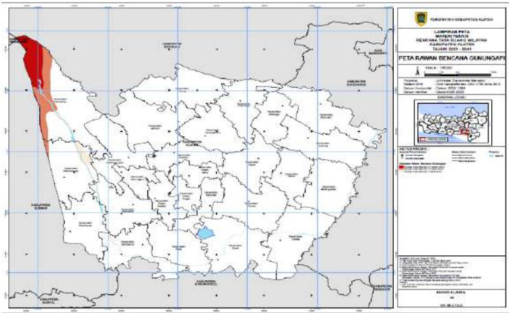
Gambar 2.64 Peta Kawasan Gunung Api di Kabupaten Klaten
